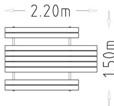
Picnic Table Olvon
